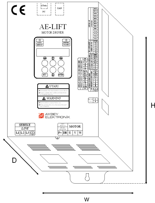
Abb. 2.1 Gehäuse „AE-LIFT“
