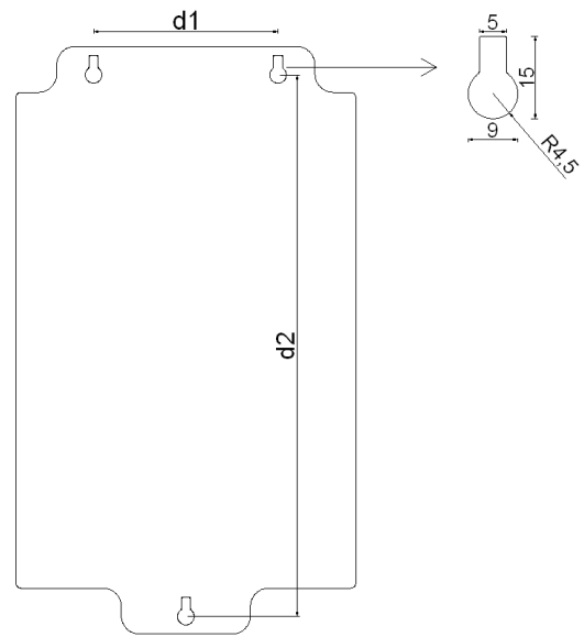
Abb. 2.2 Montagelöcher
