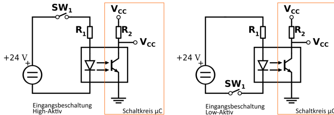
Abbildung 3-1 Erklärung der Eingangsbeschaltung anhand von Schaltbildern
