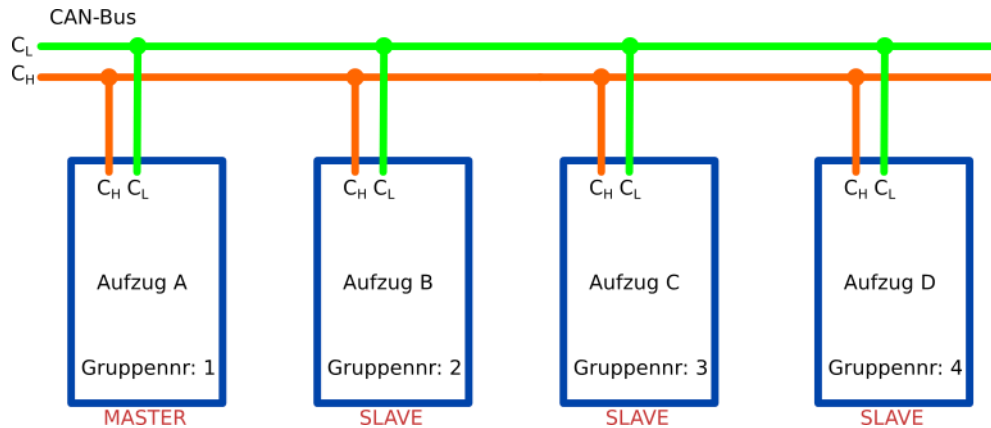
Abbildung 8-1 Veranschaulichung des ALC-Gruppenbetriebs
