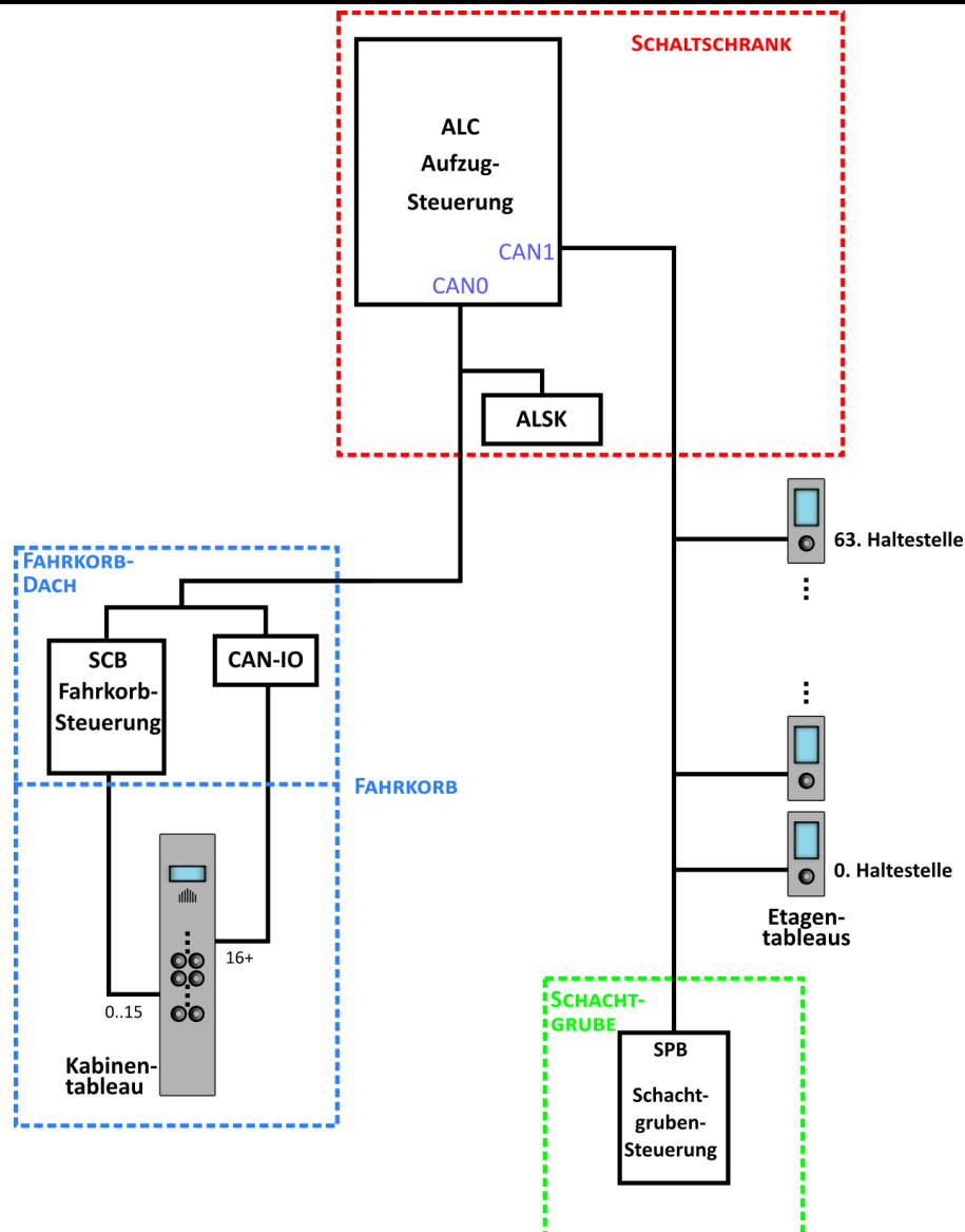
Abbildung 1-5 Alle Tableaus des Systems kommunizieren seriell über CAN-Bus
