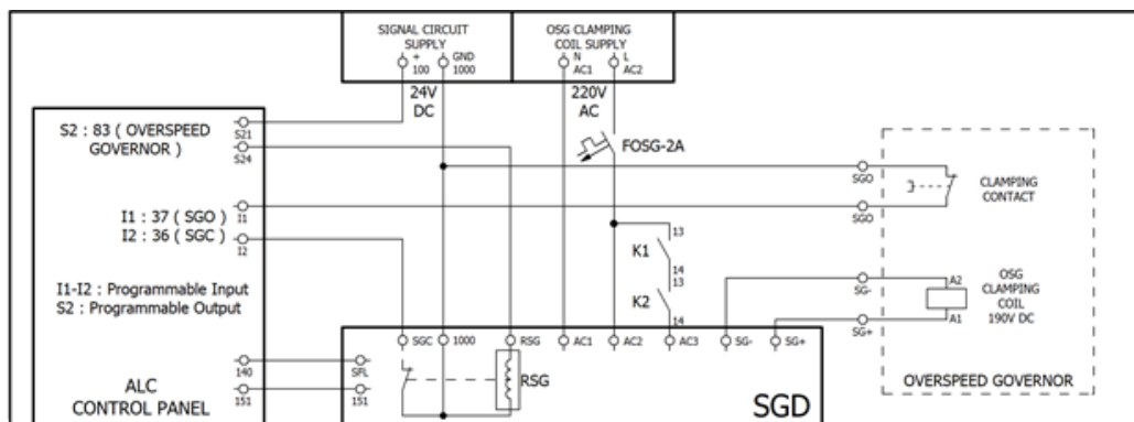
Abbildung 12-1 Schaltbild für UCM bei Traktionsaufzügen mit Asynchronmotor
