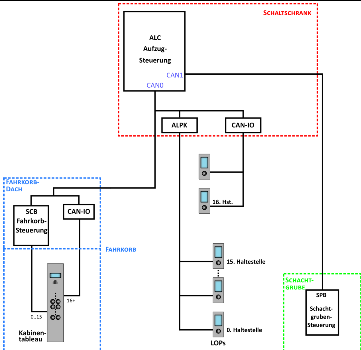
Abbildung 1-6 Im Betriebsmodus "Fahrkorb seriell" sind die Etagentableaus parallel angeschlossen.
