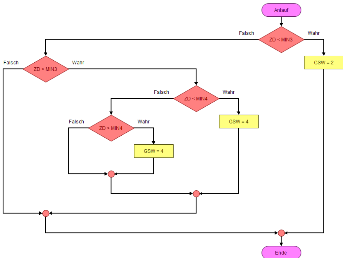
Abbildung 10-2 Entscheidung welche Geschwindigkeit die Zielgeschwindigkeit ist.
