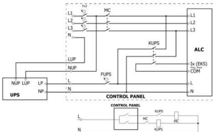
Abbildung 13-2 Schaltbild für Evakuierungssystem des Typs N
