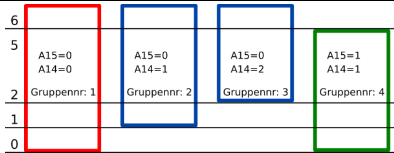
Abbildung 8-2 Der Einsatz der Parameter [A14] und [A15] bei unterschiedlicher Etagenanzahl
