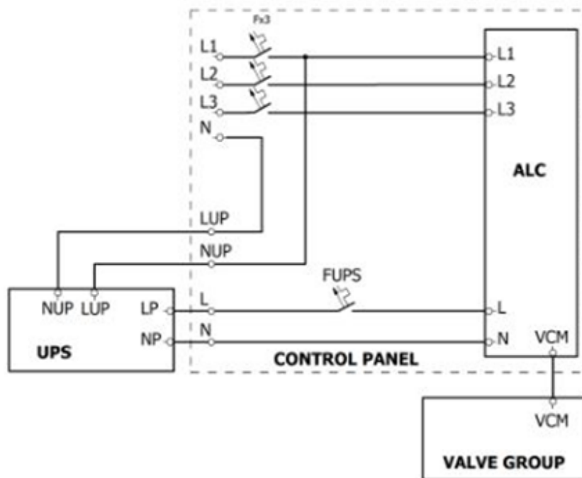
Abbildung 13-3 Schaltbild für Evakuierungssystem des Typs C
