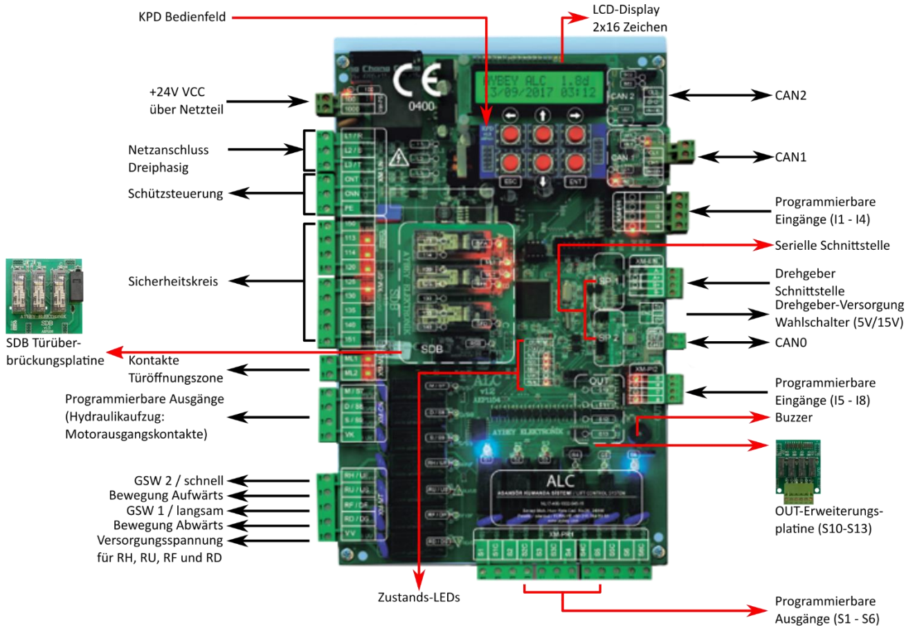
Abbildung 1-1 Hauptsteuerungsplatine des ALC-Systems
