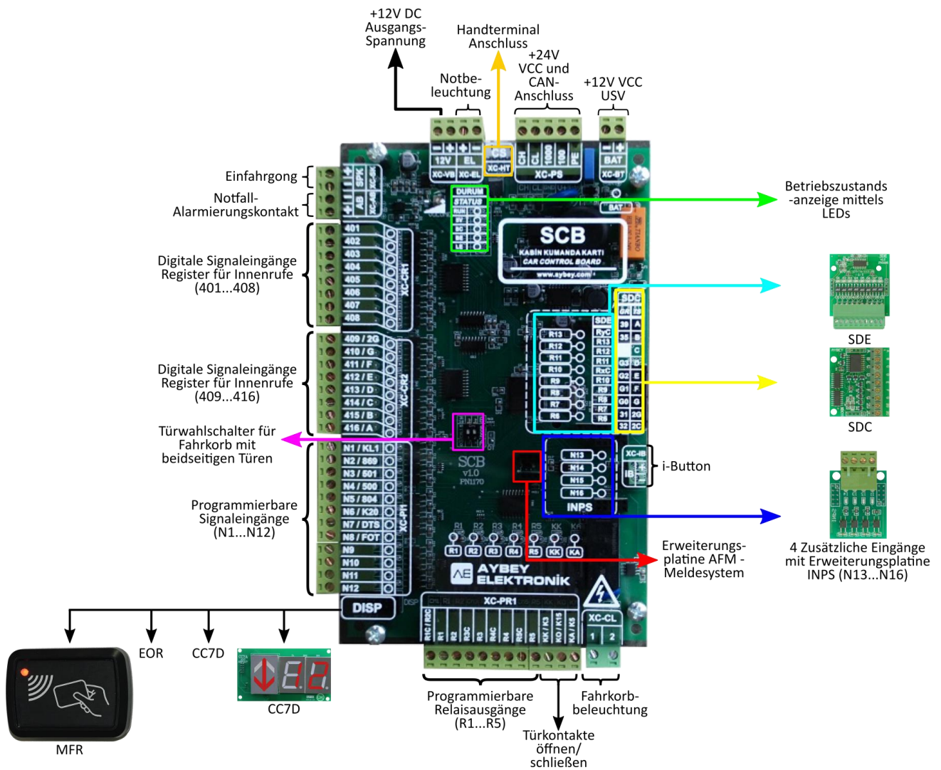
Abbildung 1-2 Die Kabinensteuerung des ALC-Systems
