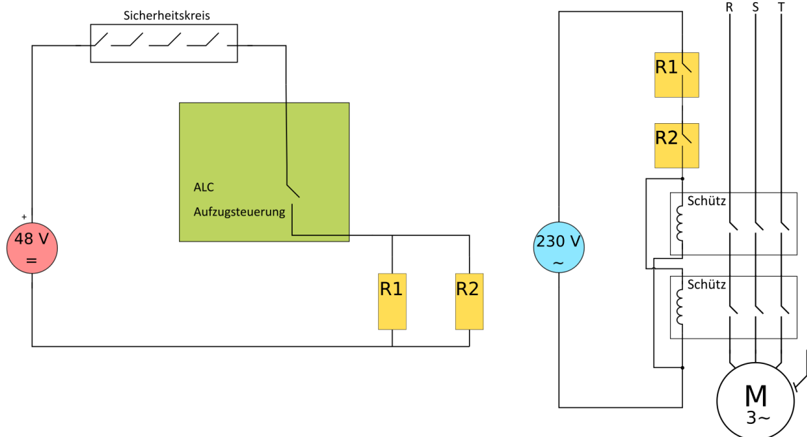
Abbildung 1-7 Beschaltung des Sicherheitskreises
