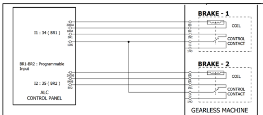
Abbildung 12-2 Schaltbild für UCM bei Traktionsaufzügen mit Synchronmotor
