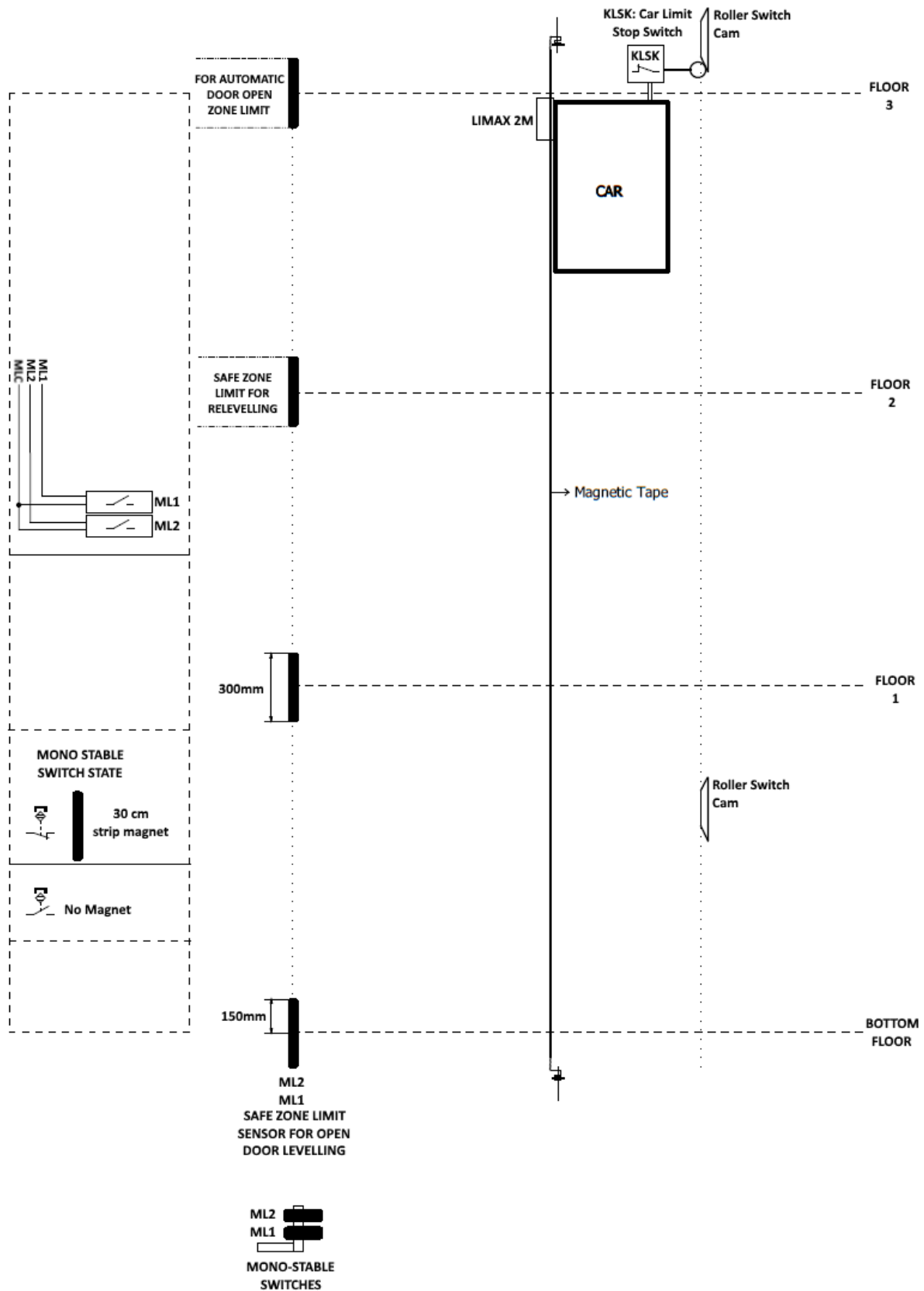
Abbildung 10-1 Platzierung der Magnete eines Absolutwertgebersystems (Limax2M)
