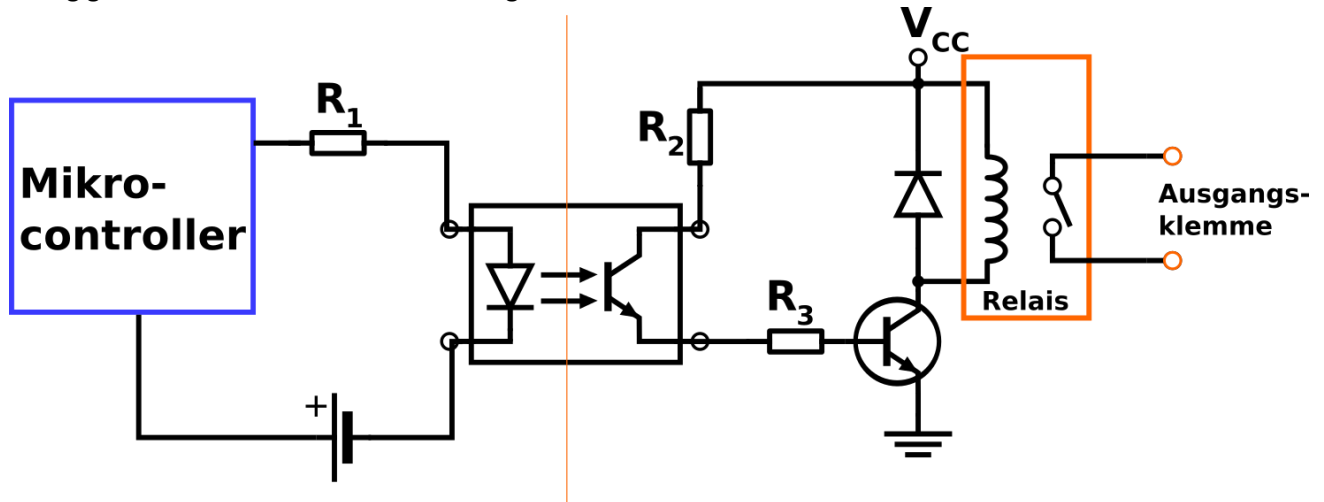
Abbildung 4-1 Ausgangsbeschaltung des ALC
