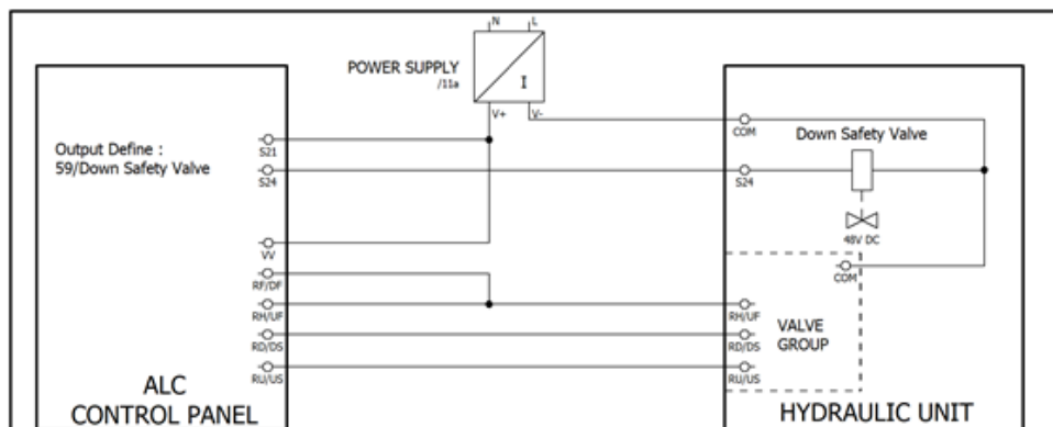
Abbildung 12-3 Schaltbild für UCM bei Hydraulikaufzügen
