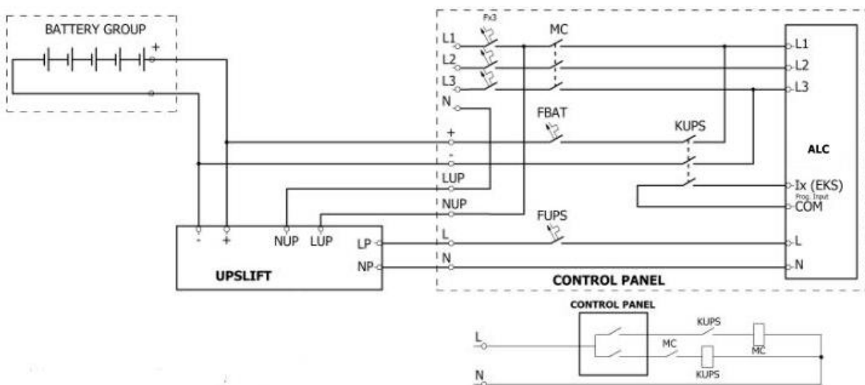
Abbildung 13-1 Schaltbild für Evakuierungssystem des Typs J
