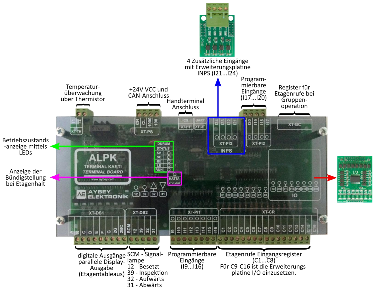
Abbildung 1-4 Die Etagentableau-Steuerung für parallel angebundene Tableaus
