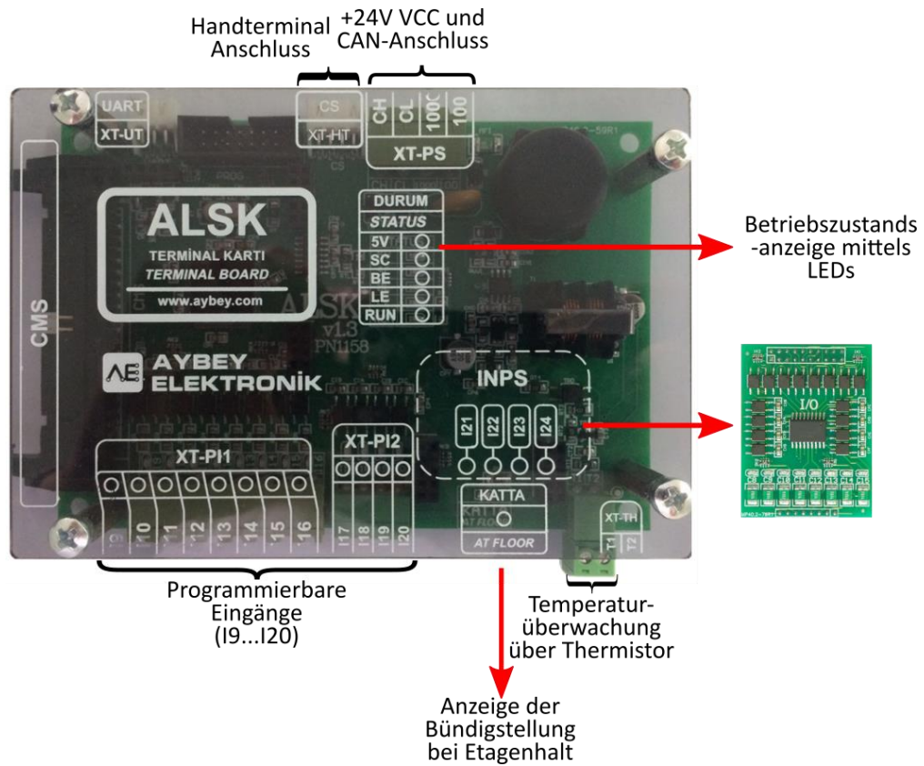
Abbildung 1-3 Die Etagentableau-Steuerung für seriell Angebundene Tableaus
