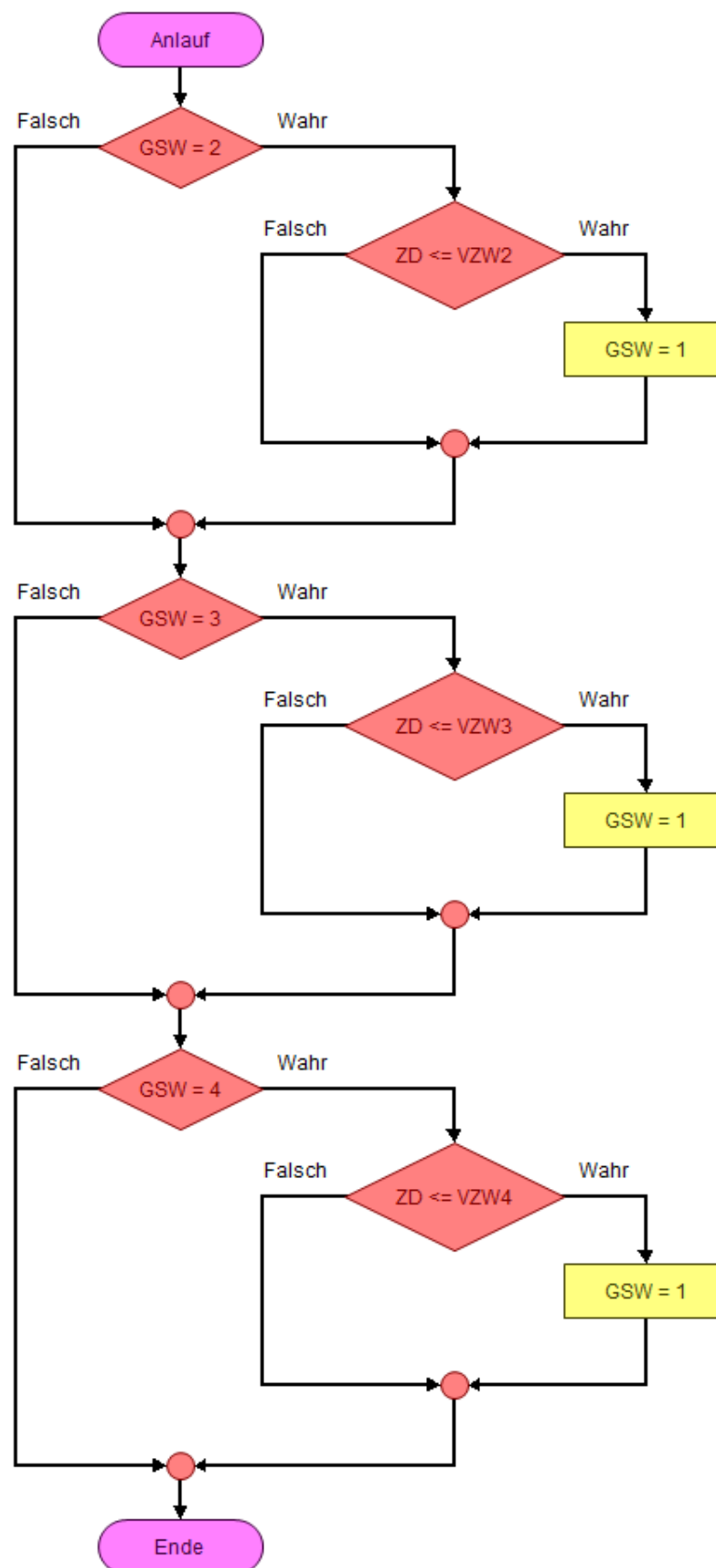
Abbildung 10-3 Entscheidungsprozess zur Verzögerung des Fahrkorbs
