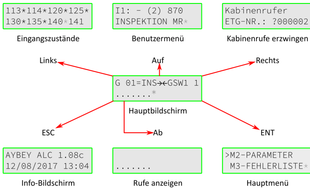
Abbildung 2-11 Beschreibung der Menüführung mittels Bedienfeld.
